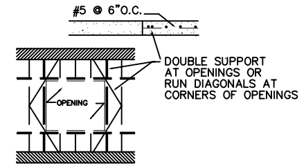
METER PIT DOOR DETAIL A
